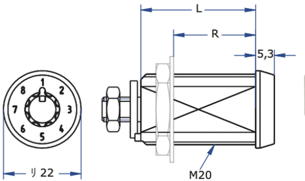
CERRADURA PROGRAMABLE
