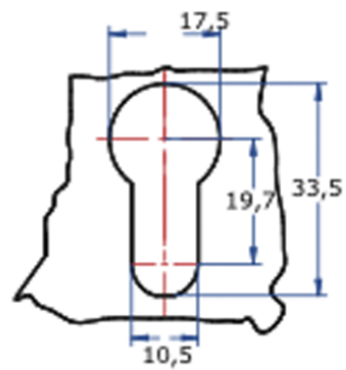
Dimensiones del orificio
