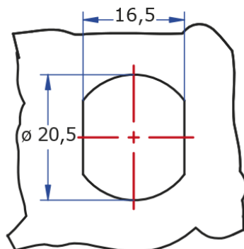
Dimensiones de orificio del bombillo
