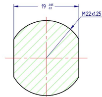
SECCION A-A 2:1
