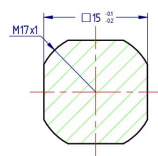
SECCION B-B 2:1
