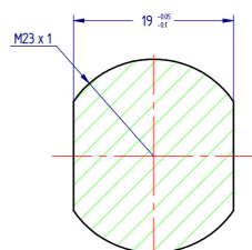
SECCION A-A 2:1
