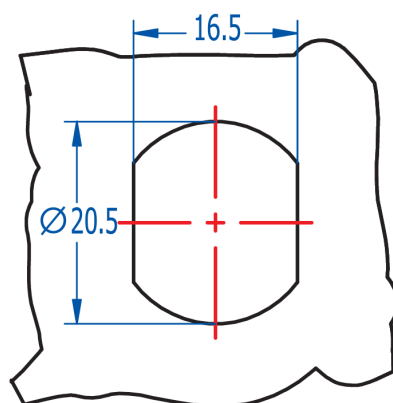
Dimensiones del orificio
