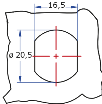
Dimensiones de orificio del bombillo
