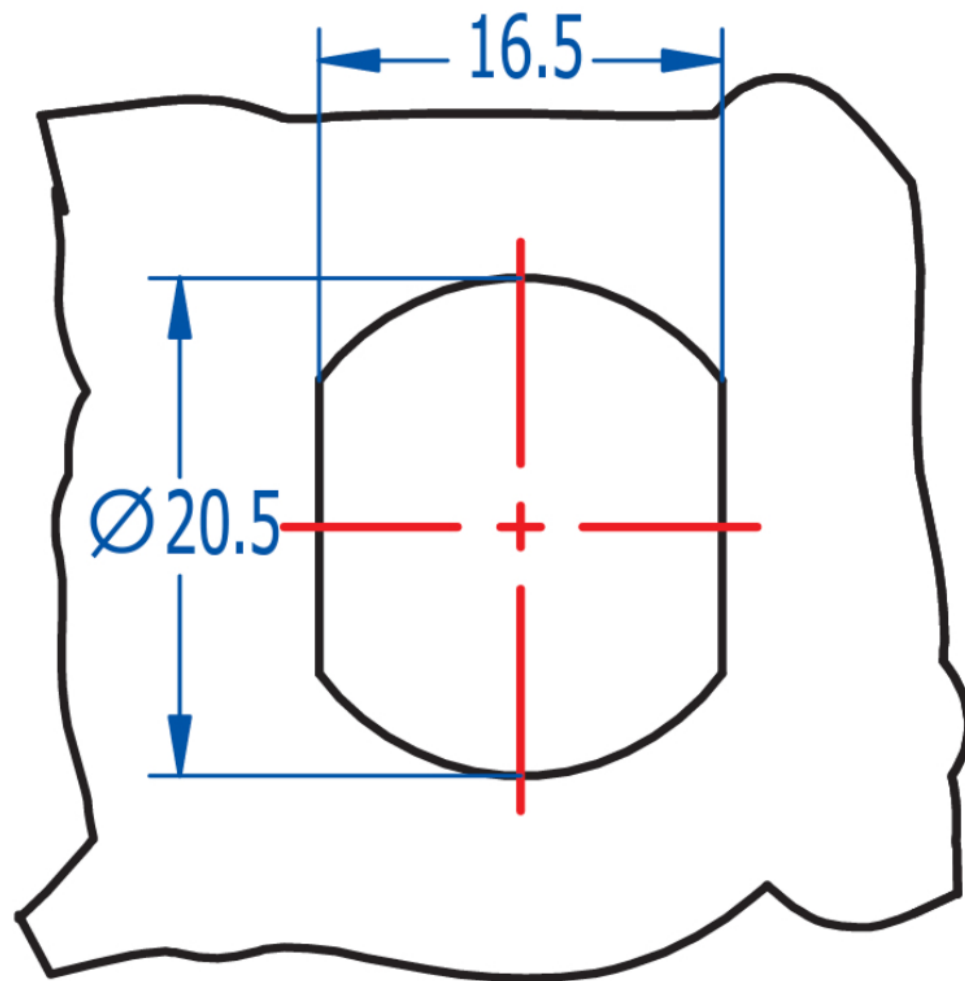
Dimensiones del orificio
