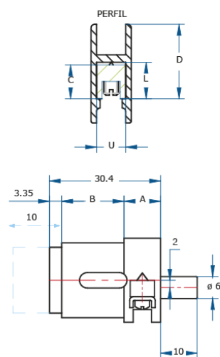
La cerradura izquierda con el croquis simétrico.
