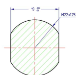
SECCION A-A 2:1
