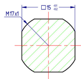
SECCION B-B 2:1
