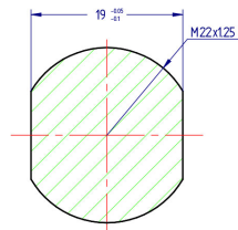
SECCION A-A 2:1
